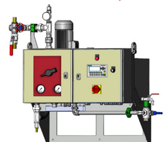
Misch- und Versorgungsstation
